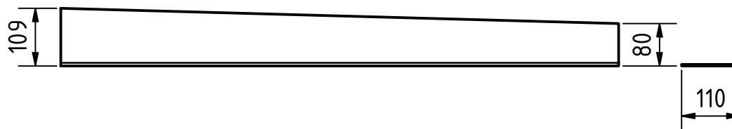
NDV-2102 Коллектор верх, s=3.0 1 шт. на NDV-2000; 4 шт. на проект
