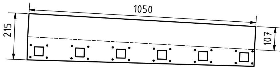
NDV-2101 Коллектор низ, s=3.0 1 шт. на NDV-2000; 4 шт. на проект
