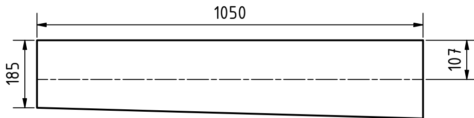
NDV-2101 Коллектор низ, s=3.0 1 шт. на NDV-2000; 4 шт. на проект
