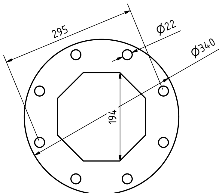
NDV-1103 Фланец центра нижний, s=5.0 1 шт. на NDV-1000; 1 шт. на проект
