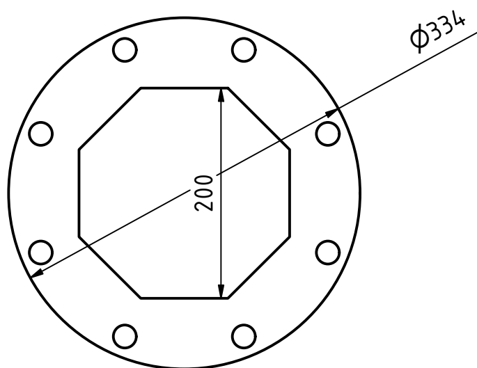
NDV-1104 Фланец центра верхний – 1 шт. на проект
